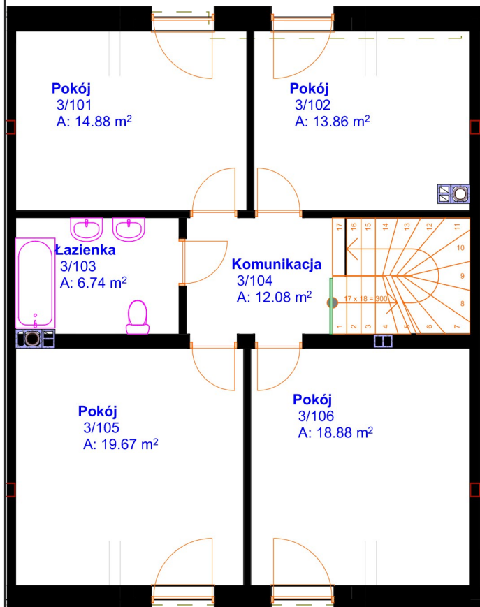
Rzut poddasza
