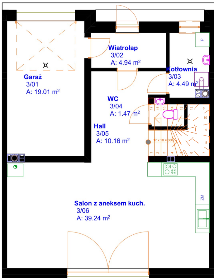
Rzut parteru
