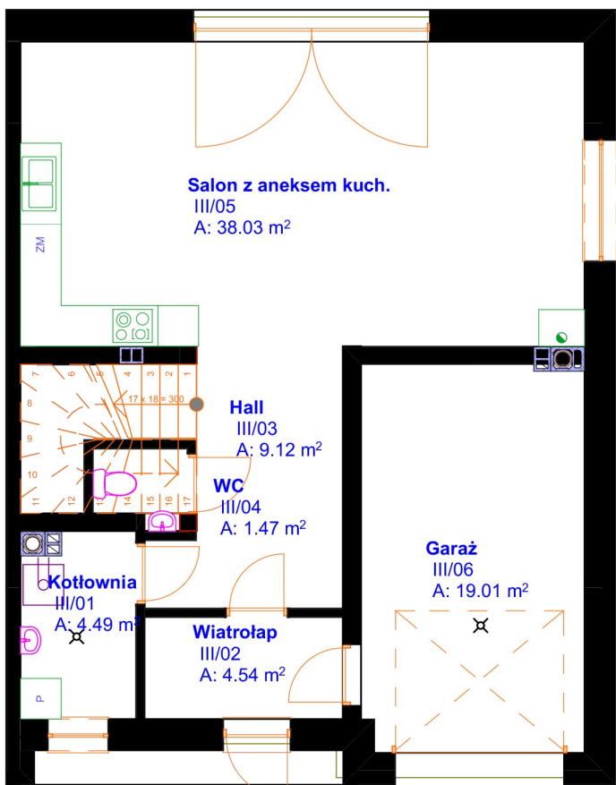
Rzut parteru
