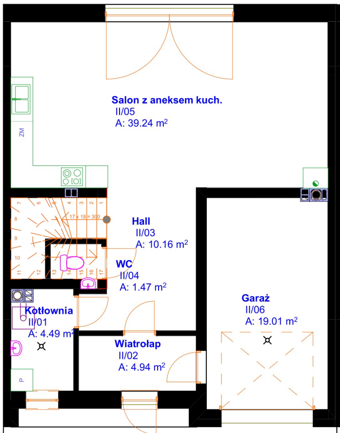
Rzut parteru
