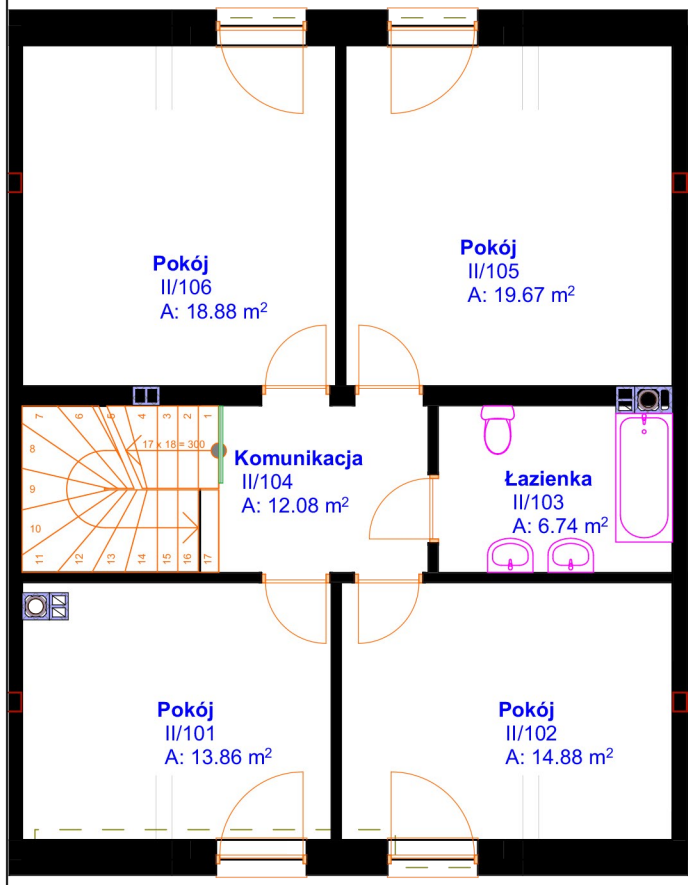
Rzut poddasza
